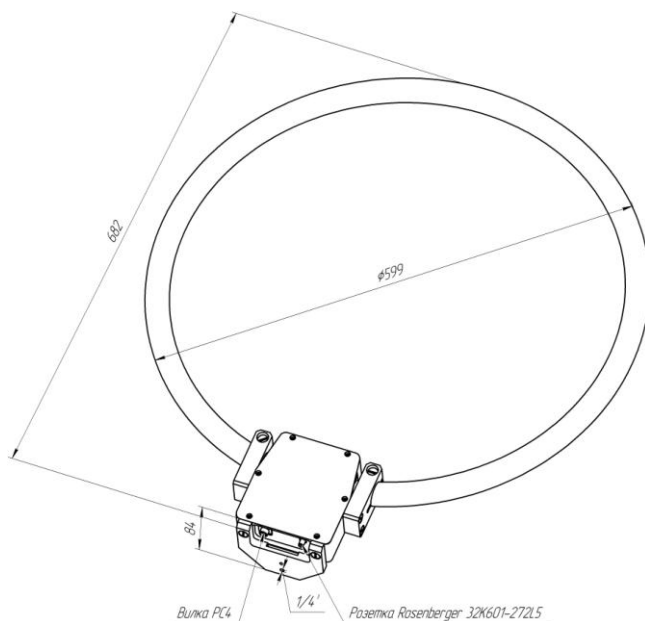
Рис.1 Габаритный чертеж антенны П6-119
