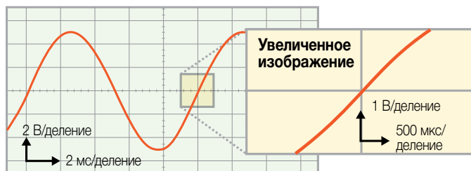
Рисунок 11б. Синусоидальный сигнал 100 Гц, сгенерированный источником B2961A/B2962A
