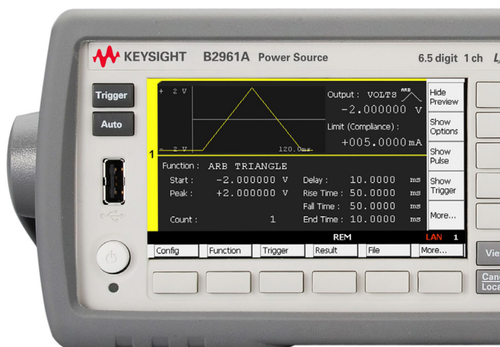
Рисунок 12. Просмотр только что созданного сигнала
