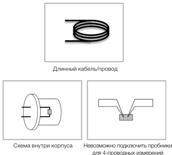
Рис. 13. Ситуации, когда удобно воспользоваться режимом программирования постоянного выходного сопротивления
