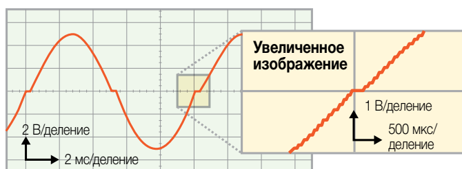
Рисунок 11а. Синусоидальный сигнал 100 Гц, сгенерированный обычным источником напряжения
