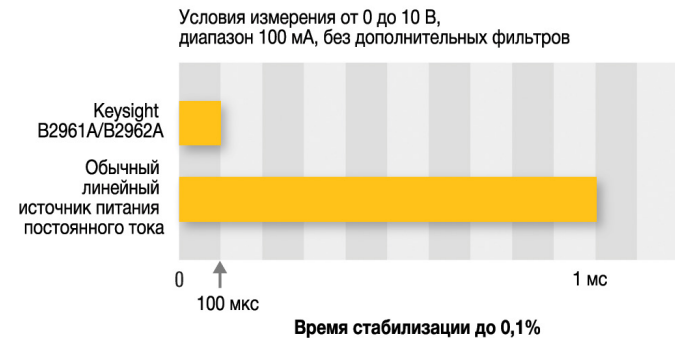
Рисунок 3. Более короткое, чем у обычных источников питания постоянного тока, время установления
