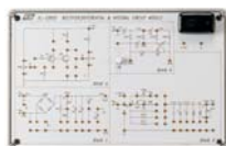
KL-23002 Схемы выпрямителя, дифференциатора и интегратора
